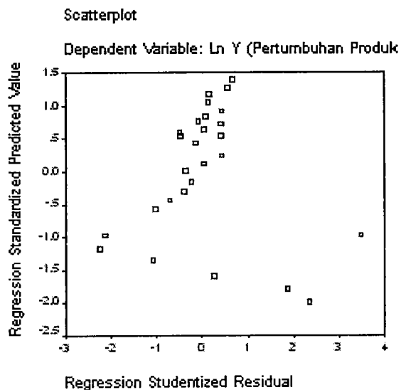
Gambar 4.2 Diagram Pencar dalam Uji Heteroskedastisitas
